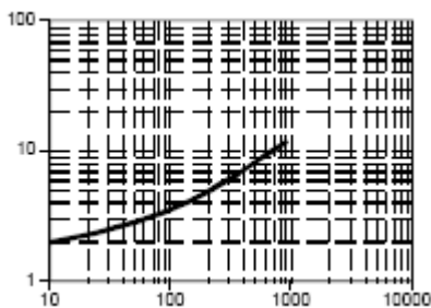
图 6. SD3443 的耦合特性
