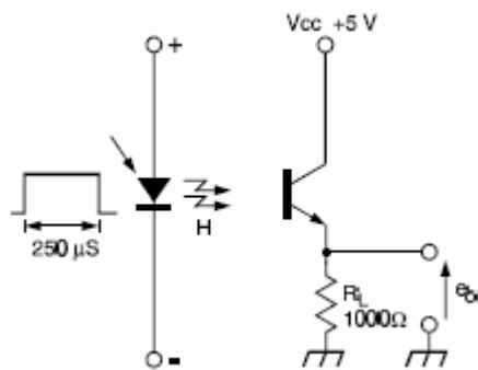
图 1 响应度与角度偏置 (SD3443) 的关系
